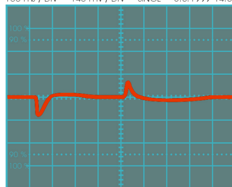
Typická odezva na změnu zátěže o 50%
